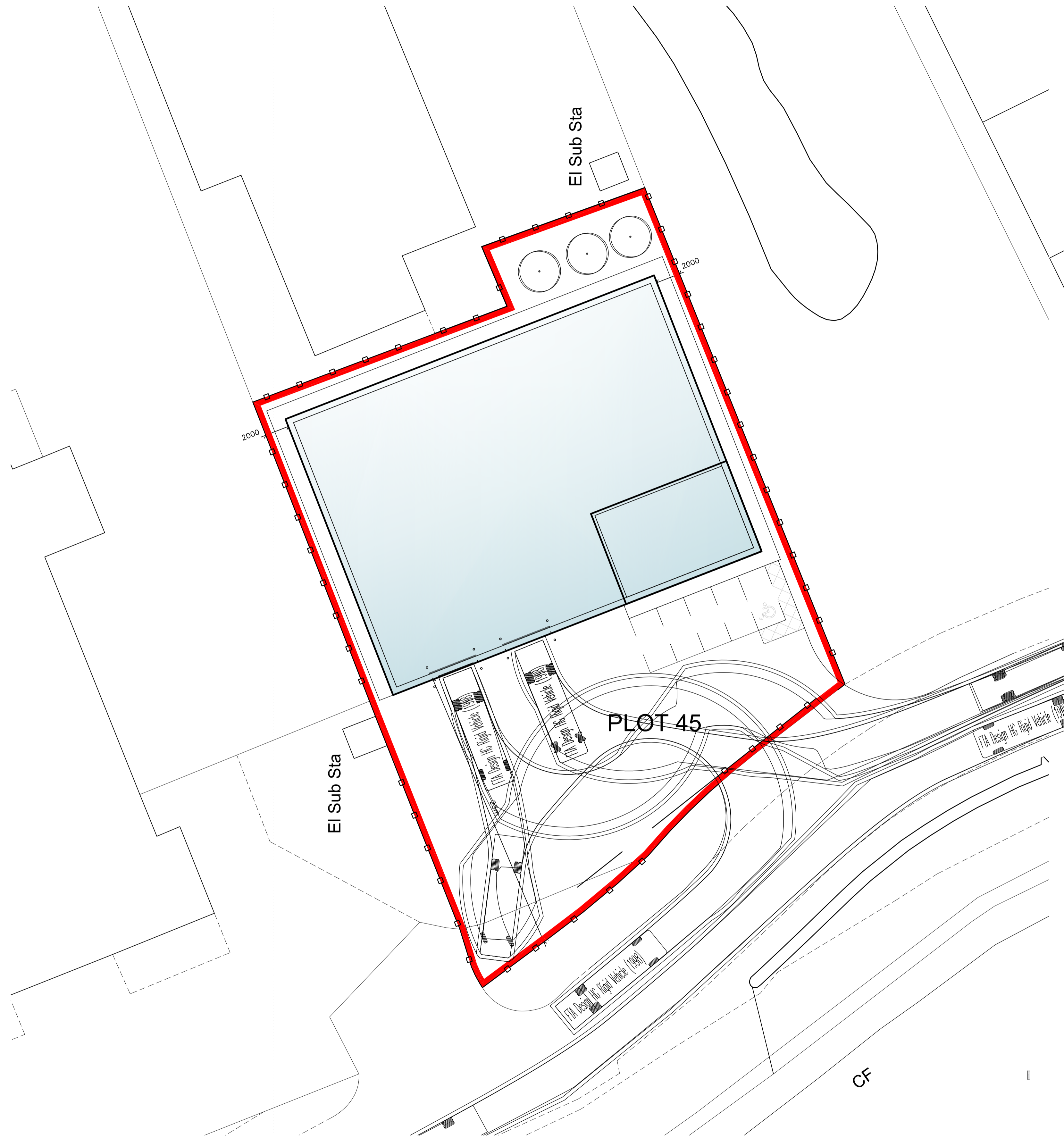
01 SITE LAYOUT PLAN 31 1:200
